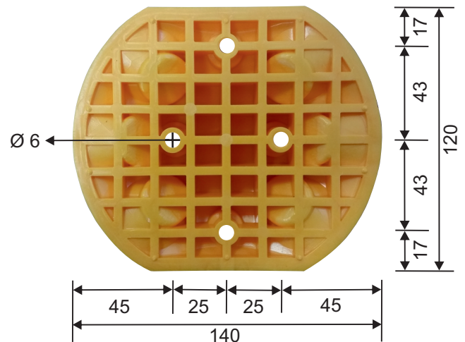
Unterseite underside
